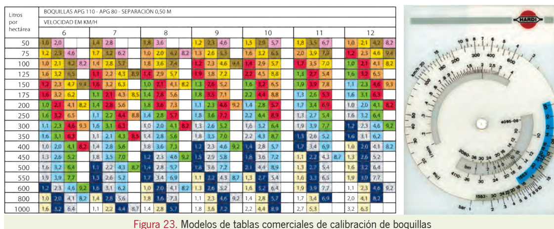
Figura 23. Modelos de tablas comerciales de calibración de boquillas
